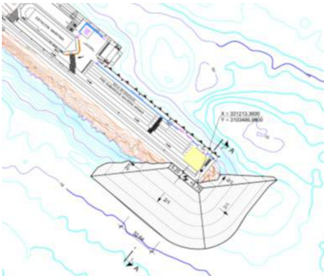
Planta de estado futuro después de la recarga del dique con bloques
