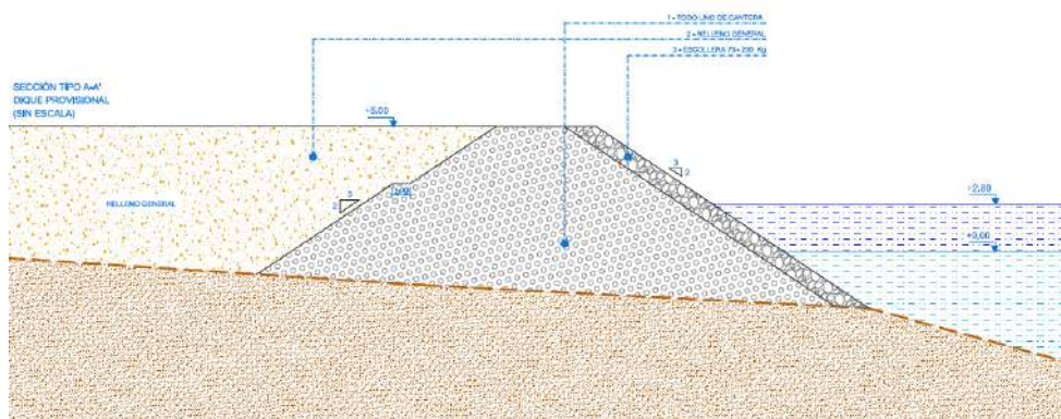
Sección tipo del dique proyectado.
