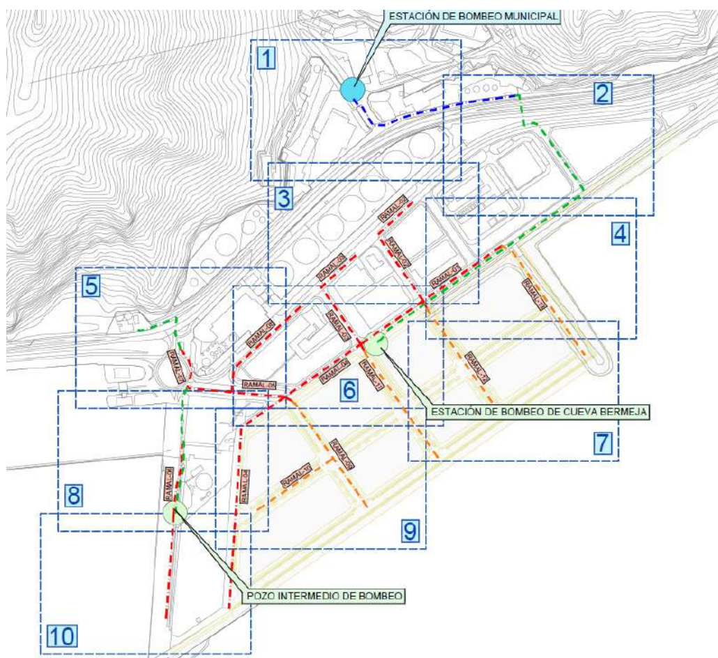
Planta General de las Obras.
