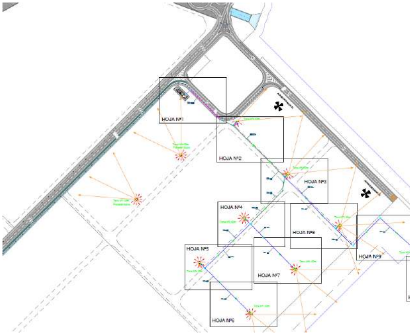
Planta de las obras.
