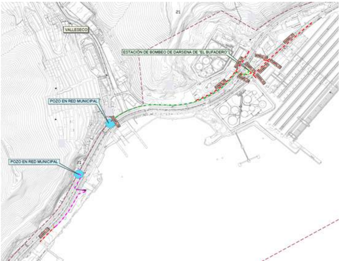
Imagen.- Planta general de las obras
