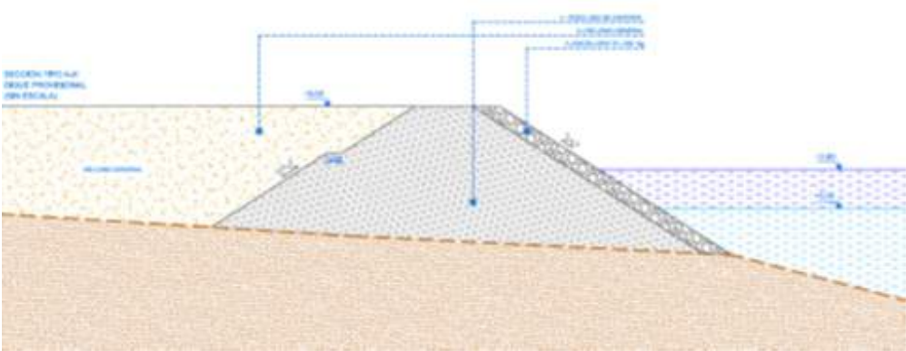
Sección tipo del dique proyectado.
