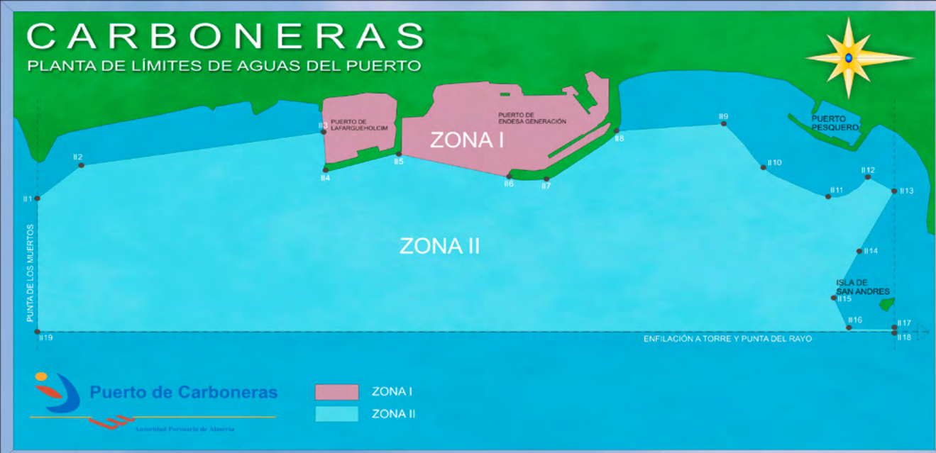
Planta de límite de aguas del puerto
