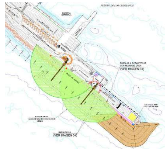
Posiciones de la grúa
