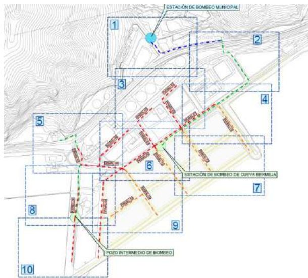
Planta General de las Obras.
