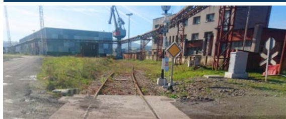
Señalización instalada a pie de vía / Signage installed at track level
