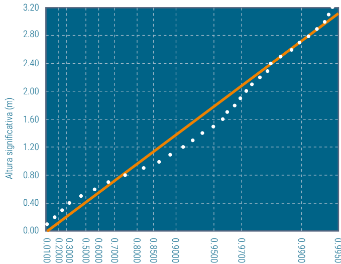
REGIMEN MEDIO DE ALTURA SIGNIFICATIVA LUGAR / Mar de Alborán SERIE / Feb 1997 - Feb 2006 PERIODO / Anual Parámetros: A = 0.62 B = -0.02 C = 1.03 < Fig 3: Régimen medio de altura de ola significante en la Boya Mar de Alborán (fuente: Organismo Público Puertos del Estado)
