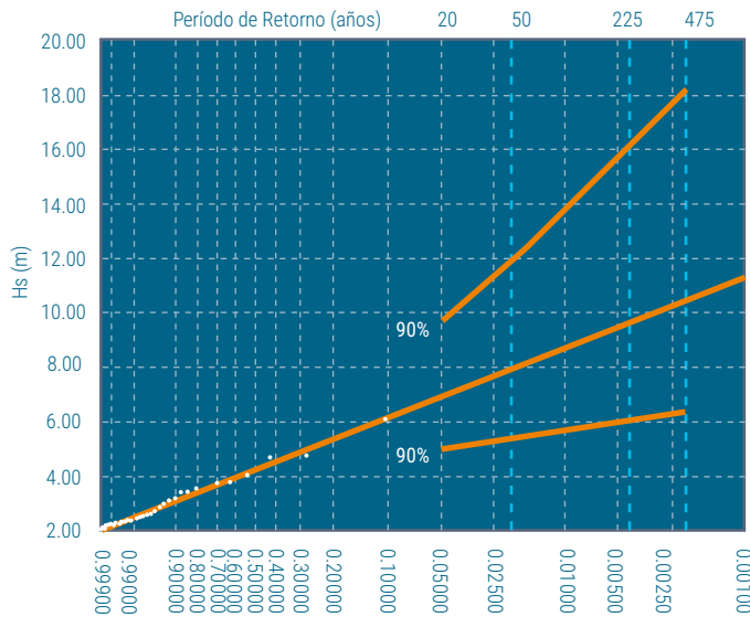
LUGAR / Mar de Alborán PARÁMETRO / Altura Significante PROFUNDIDAD / 530.0 SERIE ANALIZADA / Jun 1997 - Nov 2005 < Fig 4: Régimen extremal escalar de altura de ola significante en la Boya Mar de Alborán
