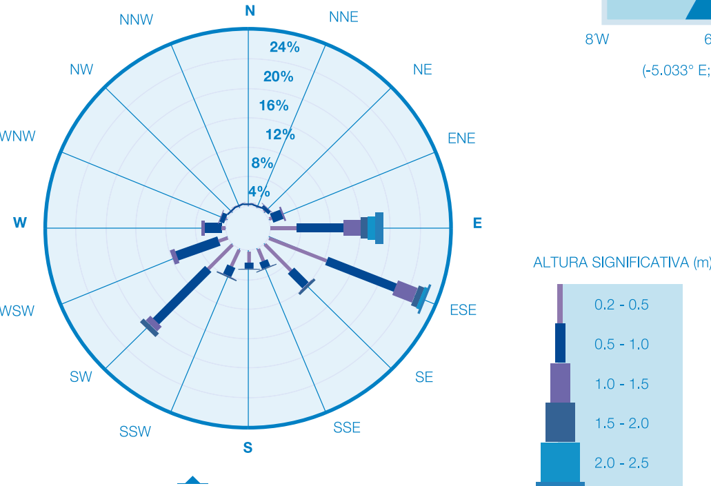
FIG 2: ROSA DE OLEAJE BOYA MAR DE ALBORÁN. (Fuente: Organismo Público Puertos del Estado)
