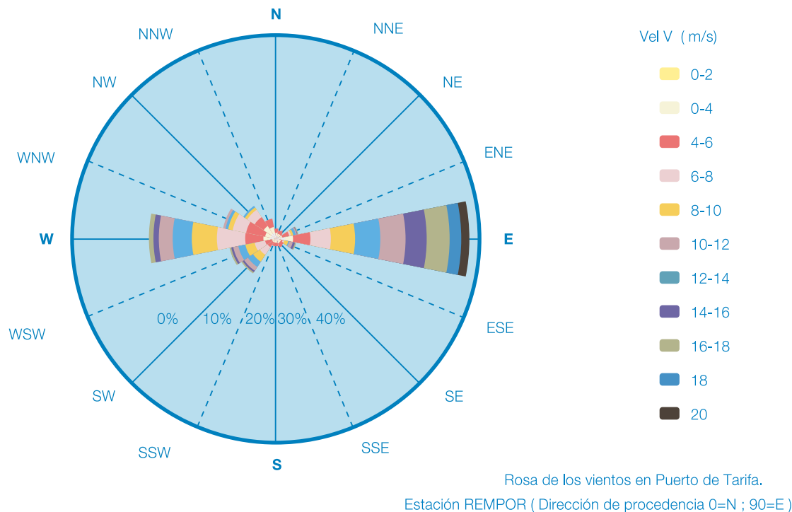
ROSA DE VIENTOS Estación Puerto de Tarifa
