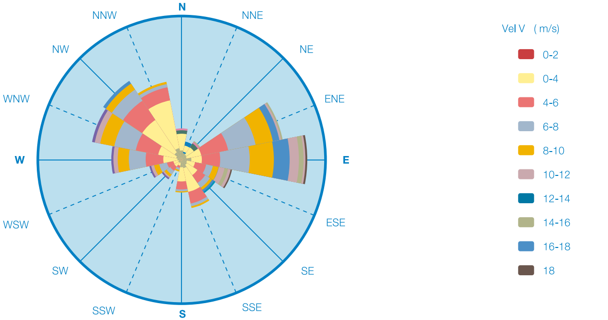
Rosa de los vientos en Puerto de Algeciras. Estación REMPOR ( Dirección de procedencia 0=N ; 90=E )
