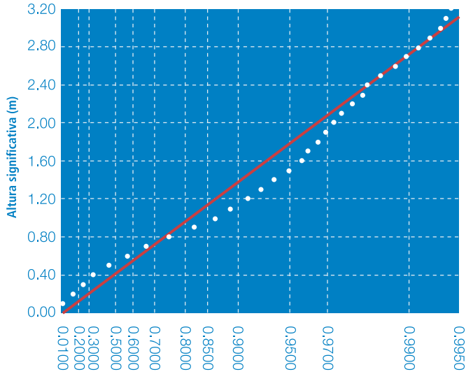
REGIMEN MEDIO DE ALTURA SIGNIFICATIVA
