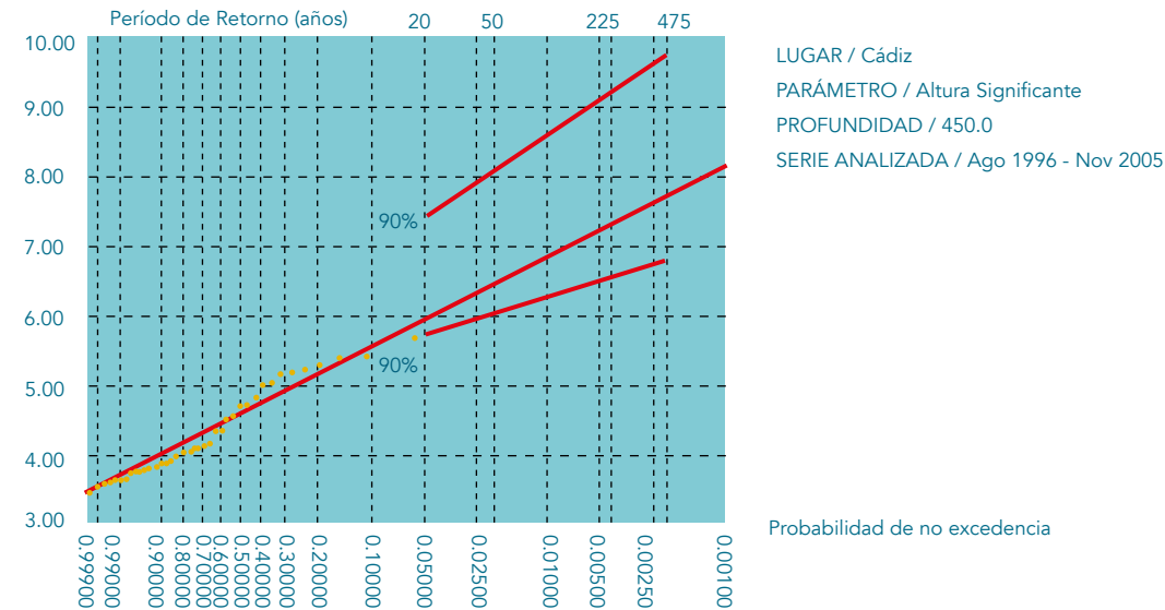
← Fig 10: Régimen extremal escalar de altura de ola significativa en la Boya Golfo de Cádiz
