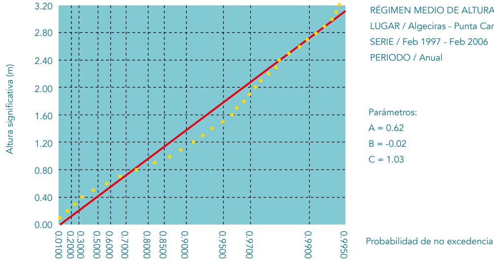
Fig 4: Régimen medio de altura de ola significativa en la Boya de Algeciras - Punta Carnero (Fuente: Organismo Público Puertos del Estado)
