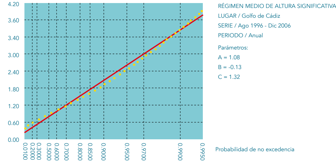
← Fig 9: Régimen medio de altura de ola significativa en la Boya de Golfo de Cádiz. (Fuente: Organismo Público Puertos del Estado)
